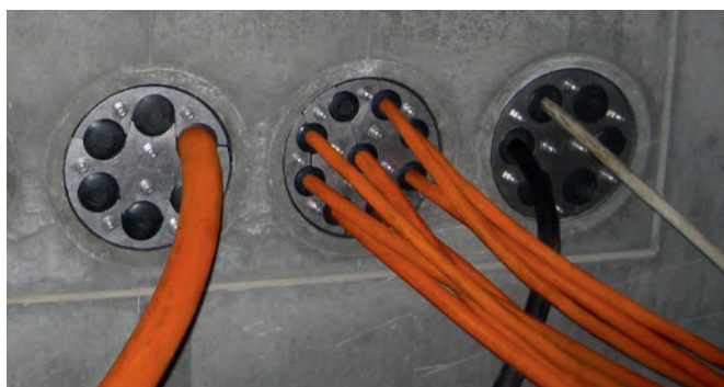
HRD 150-SG – monté dans des fourreaux fibrociment
